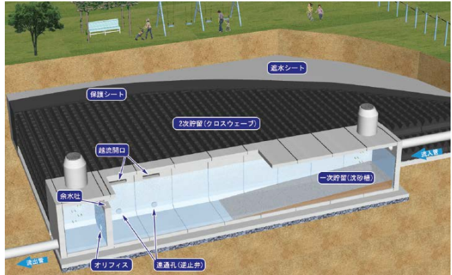
複合型雨水貯留システム「ダブルポート」
